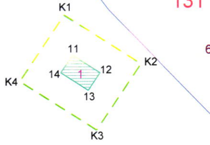
1-ITRF96-45/3 Derece
