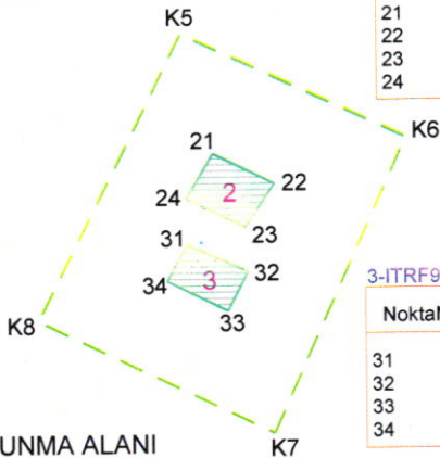
2-ITRF96-45/3 Derece
